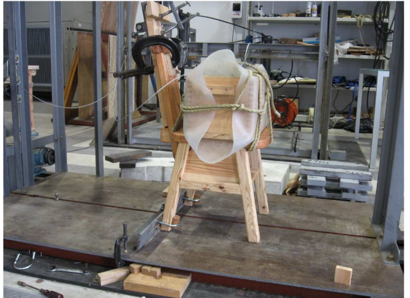
椅子の耐久性強度試験
